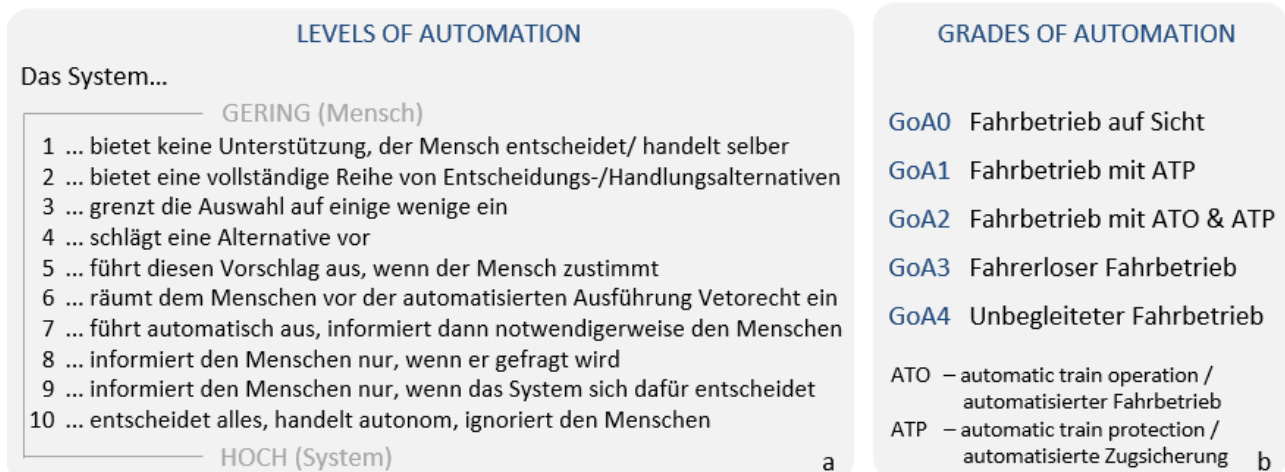
Abb. 2: a) Automatisierungsgrade in Bezug auf die menschliche Informationsverarbeitung (Sheridan & Verplank, 1978; Parasuraman et al., 2000) und b) Automatisierungsgrade (GoA) in Bezug auf den Zugbetrieb (Braband, 2021, UITP, 2018).
