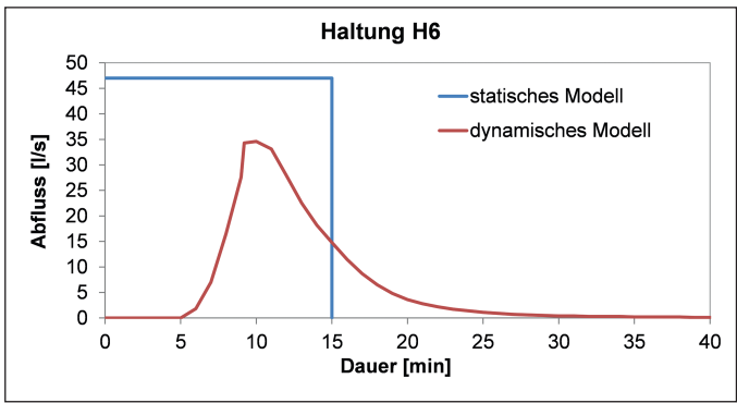
Abb. 4: Blockabfluss des statischen Modells und Abflussganglinie des dynamischen Modells am Beispiel der Haltung H6
